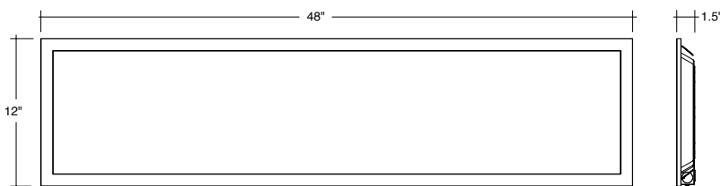
1X4
