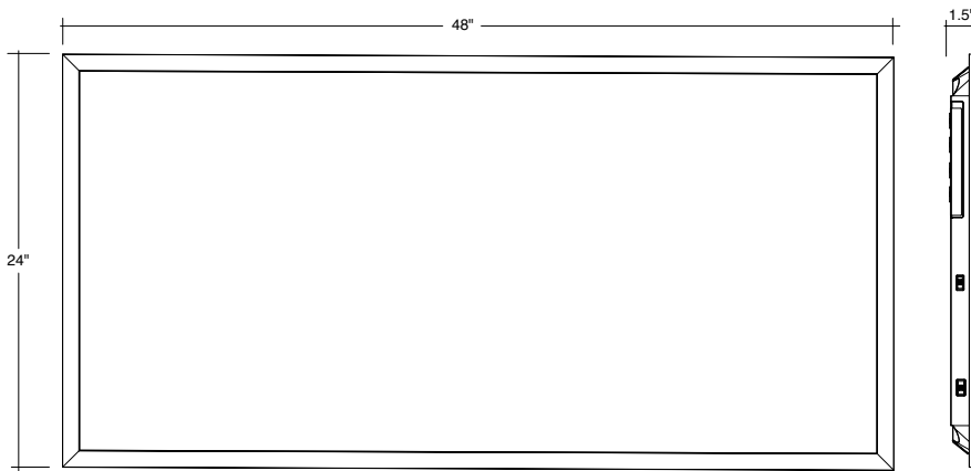
2X4
